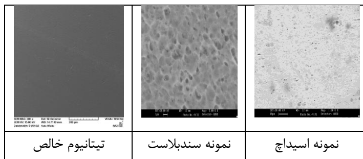
شکل ۱- نمونه وایر های مورد آزمایش پس از آماده سازی سطحی. میکروسکوپ الکترونی (SEM) بزرگنمایی ۱۰۰۰ x
